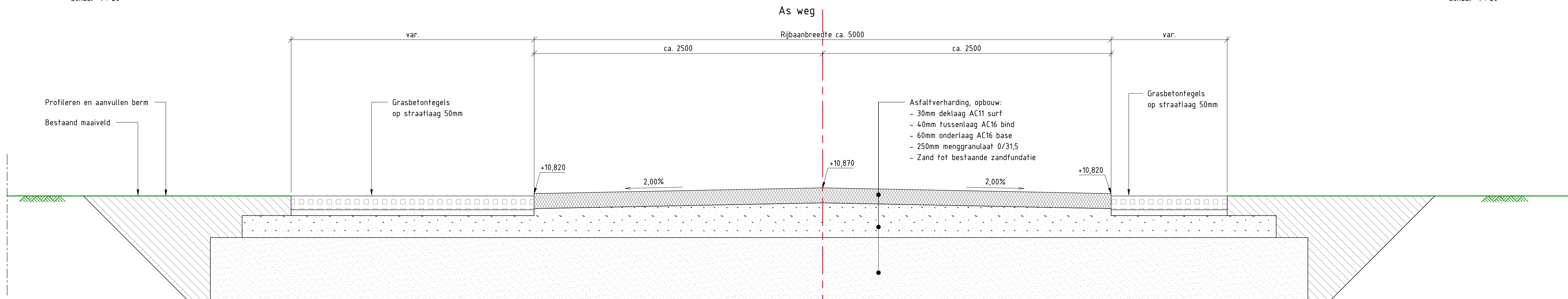
Doorsnede B-B Schaal 1 : 20
