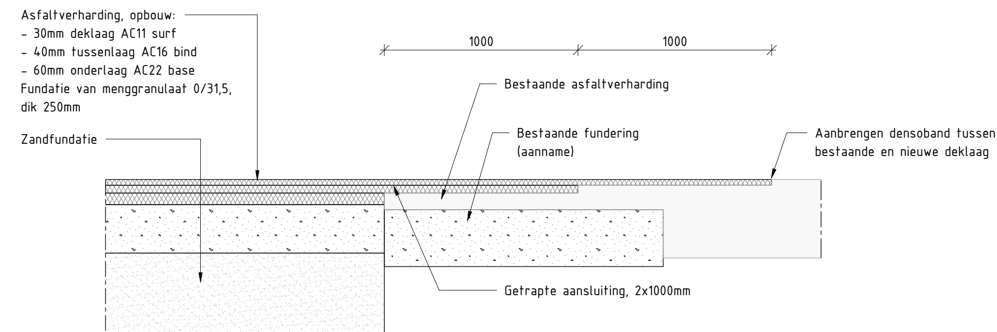
Detail - Aansluiting verharding Schaal 1 : 20
